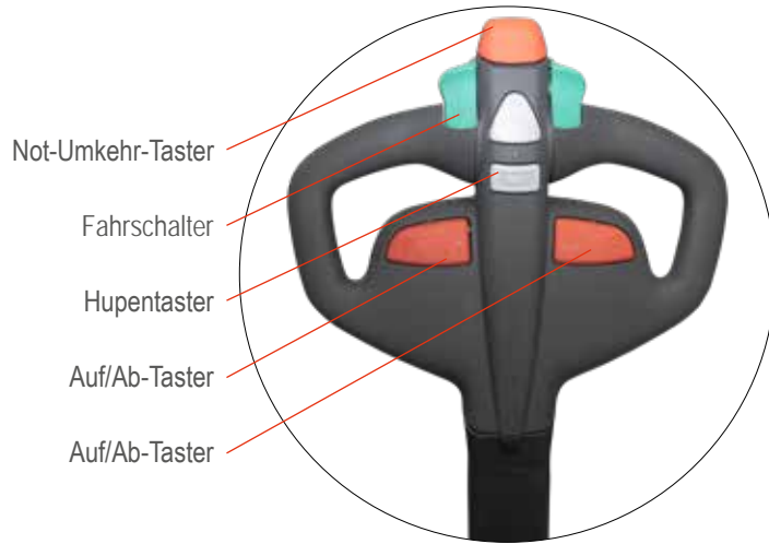
Multifunktionsgriff
